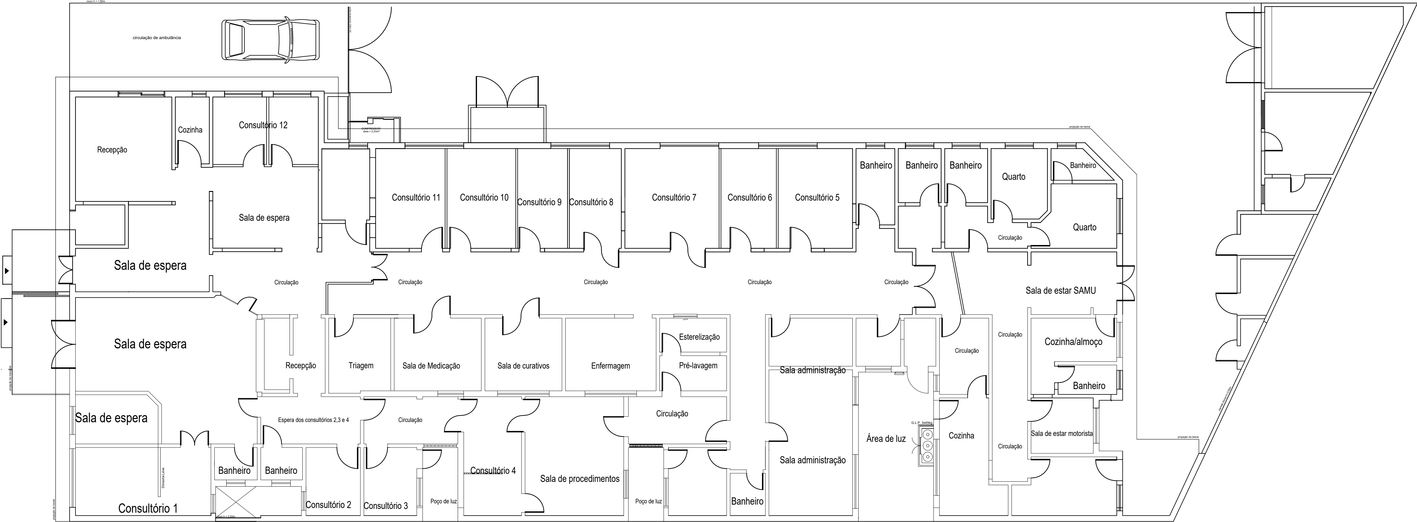
PLANTA BAIXA ESC 1/100
