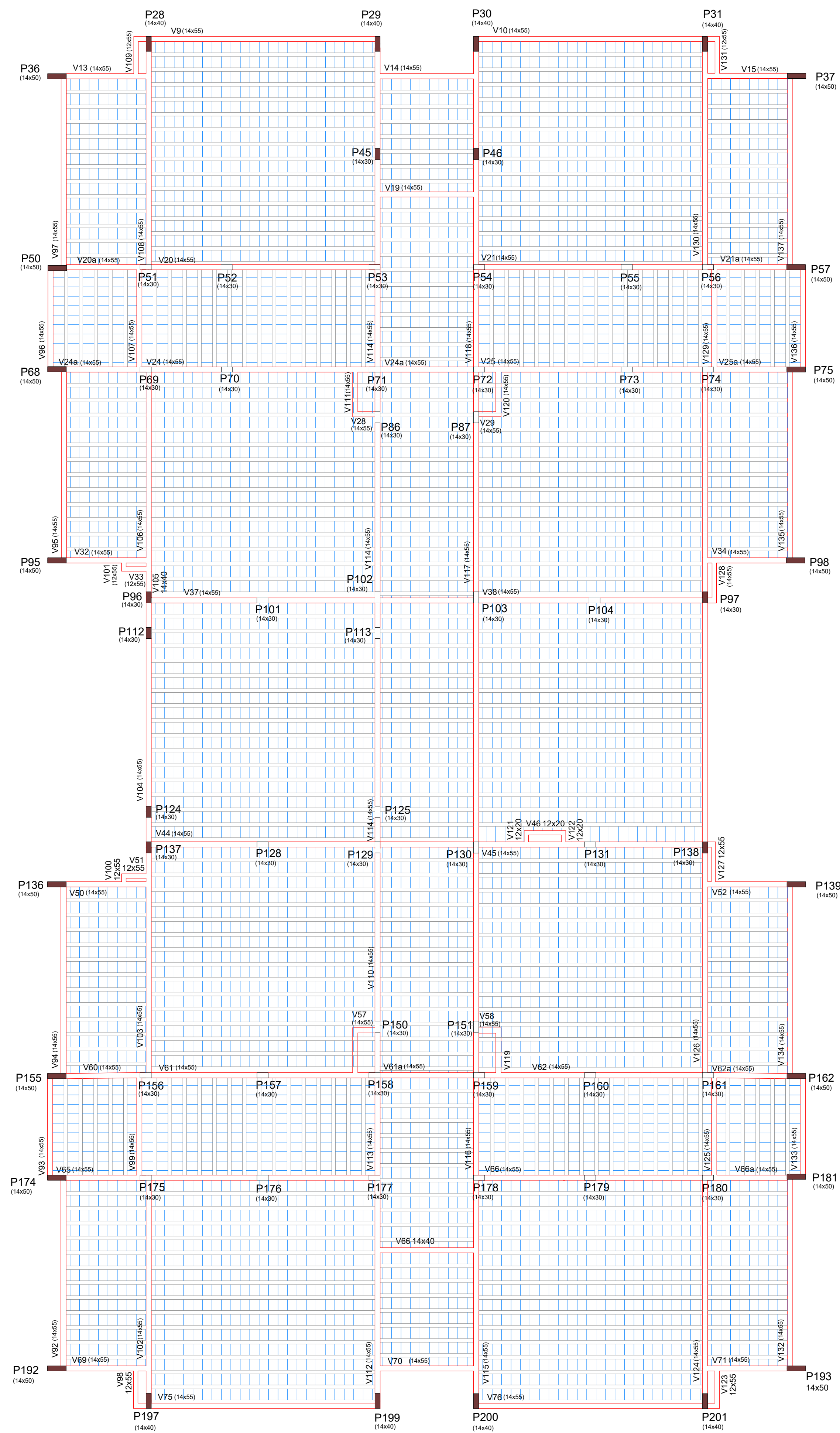
VIGAS DE COBERTURA E DISPOSIÇÃO DA LAJE PRÉ-MOLDADA
